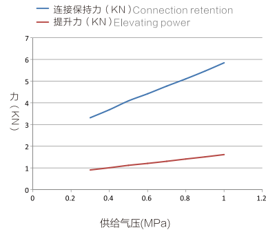
OQT-40 连接力、提升力曲线图
