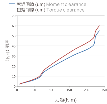
OQT-40 弯矩、扭矩变位曲线图
